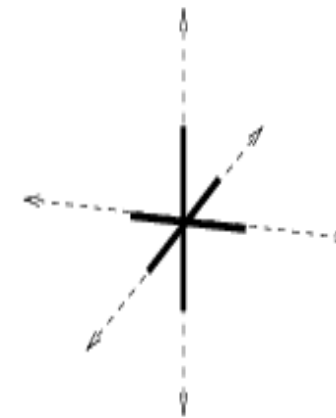
Sparse data
