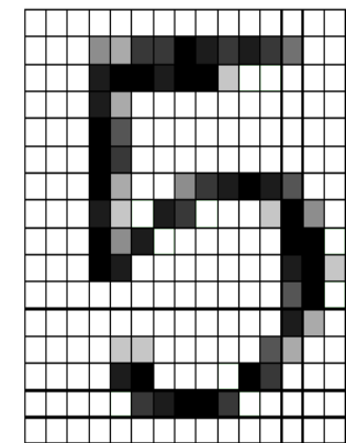
Sparse data
