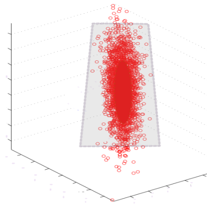
Linear data
